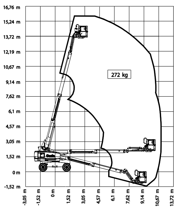
S-45 HF Diagram werkbereik
