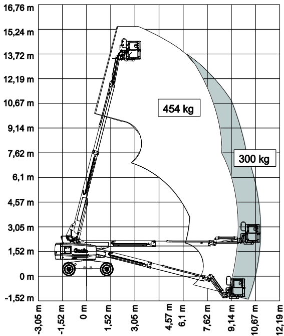
Diagram werkbereik S-45 XC en S-45 TRAX
